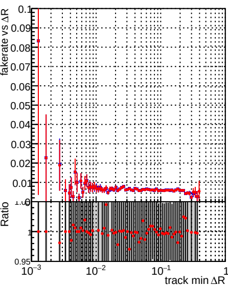
Legend: —•— DQM_TTPU_mkFit_BuildNEW3 —•— DQM_TTPU_mkFit_BuildNEW4
