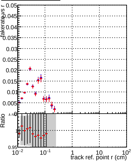
Fake rate vs vertpos DQM_TTPU_mkFit_Build DQM_TTPU_mkFit_BuildNEW3
