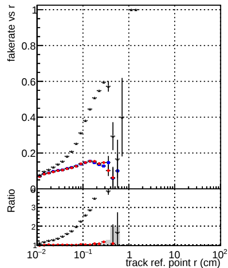
Global CKF RECO Global mkFit1 RECO Global mkFit2 RECO
