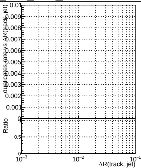
Global mkFit1 RECO Global mkFit2 RECO
