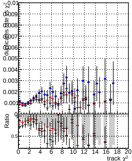
a mkFit1 REC8 a mkFit2 REC8
