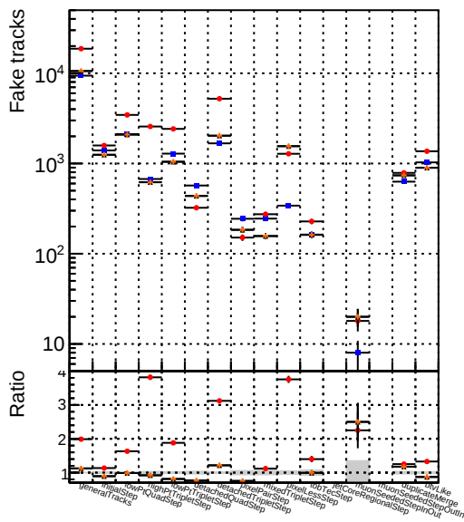
Number Legend 1 DQM_mkFit_softQCD 2 DQM_mkFit_softQCD-ncp 3 DQM_mkFit_softQCD-newTr3
