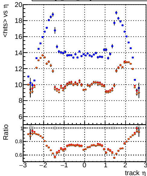
mean hit — DQM_CKF_softQCD — DQM_mkFit_softQCD — DQM_mkFit_softQCD-ncp — DQM_mkFit_softQCD-newTr3
