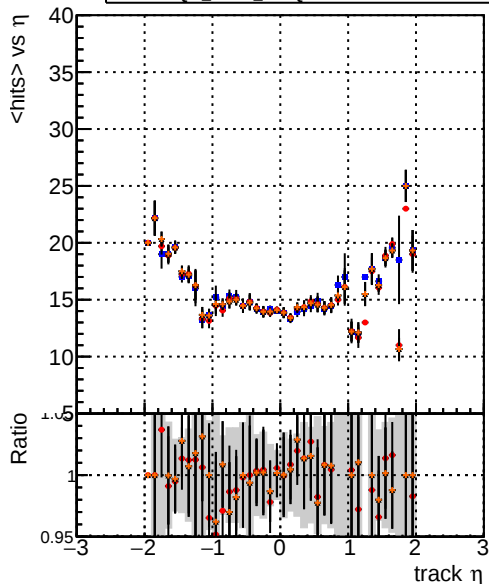
DQM_CKF_softQCD DQM_mkFit_softQCD DQM_mkFit_softQCD-ncp DQM_mkFit_softQCD-newTr3 mean hit
