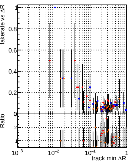
Fake rate vs \Delta R(\text{track, jet}) DQM CKF softQCD DQM mktFit softQCD DQM mktFit softQCD-np DQM mktFit softQCD-newTr3
