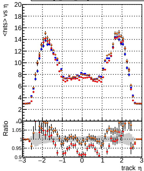
DQM_CKF_fit_softQCD DQM_mkFit_softQCD DQM_mkFit_softQCD-ncp DQM_mkFit_softQCD-newTr3 mean hit
