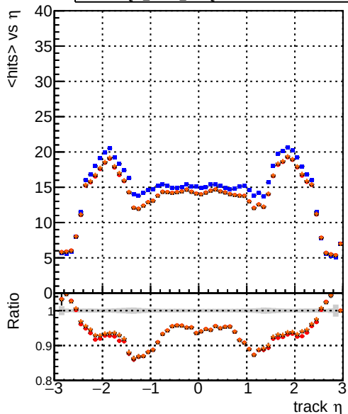
Legend: — DQM_CKF_softQCD — DQM_mkFit_softQCD — DQM_mkFit_softQCD-ncp — DQM_mkFit_softQCD-newTr3 mean hit
