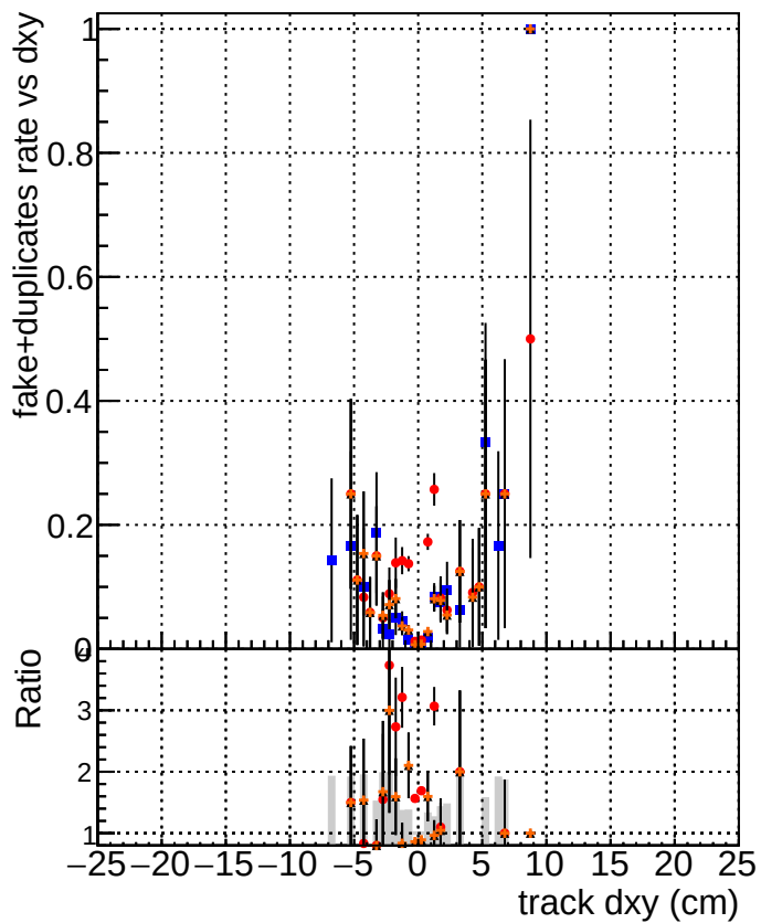
Legend for the plots: DQM_CKF_softQCD DQM_mkFit_softQCD DQM_mkFit_softQCD-ncp DQM_mkFit_softQCD-newTr3
