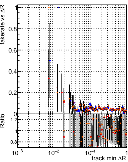
Fake rate vs \Delta R(\text{track, jet}) —●— DQM —●— CKE —●— softQCD —●— QCD —●— DQM —●— CKE —●— softQCD —●— QCD —●— DQM —●— CKE —●— softQCD —●— QCD —●— DQM —●— CKE —●— softQCD —●— QCD —●— DQM —●— CKE —●— softQCD —●— QCD —●— DQM —●— CKE —●— softQCD —●— QCD —●— DQM —●— CKE —●— softQCD —●— QCD —●— DQM —●— CKE —●— softQCD —●— QCD —●— DQM —●— CKE —●— softQCD —●— QCD —●— DQM —●— CKE —●— softQCD —●— QCD
