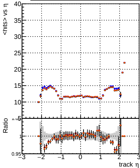
mean hit — DQM_CKF_fit_softQCD — DQM_mkFit_fit_softQCD — DQM_mkFit_fit_softQCD-ncp — DQM_mkFit_fit_softQCD-newTr3
