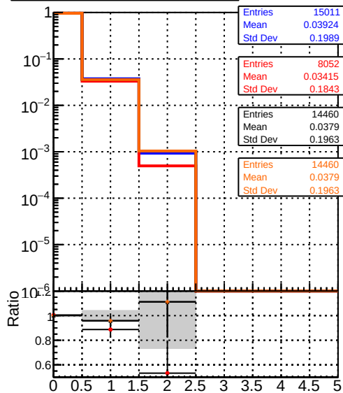
mean hit DQM_CKF_softQCD DQM_mkFit_softQCD DQM_mkFit_softQCD-ncp DQM_mkFit_softQCD-newTr3
