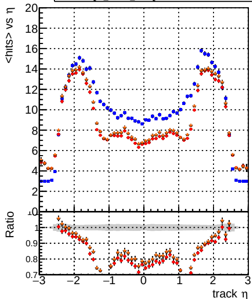
mean hit DQM_CKF_fit_softQCD DQM_mkFit_fit_softQCD DQM_mkFit_fit_softQCD-ncp DQM_mkFit_fit_softQCD-newTr3
