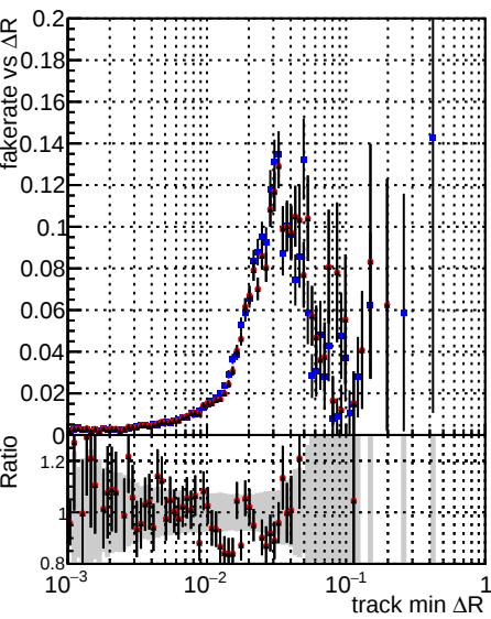
Legend: DQM_CKF_softQCD (blue circles), DQM_mkFit_softQCD (red circles), DQM_mkFit_softQCD-newTr2 (black circles)
