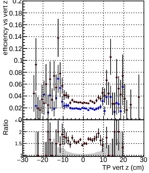
Efficiency vs. sim PV z — DQM_CKF_softQCD — DQM_mkFit_softQCD — DQM_mkFit_softQCD-newTr2
