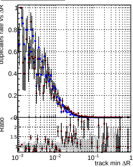
Legend: DQM_CKF_softQCD (black), DQM_mkFit_softQCD (red), DQM_mkFit_softQCD-newTr2 (blue)
