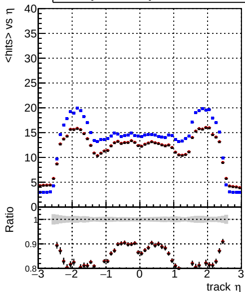
mean hit — DQM_CKF_softQCD — DQM_mkFit_softQCD — DQM_mkFit_softQCD-newTr2
