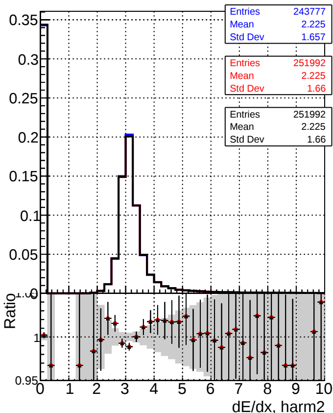
DQM_CKF_softQCD DQM_mkFit_softQCD DQM_mkFit_softQCD-newTr2
