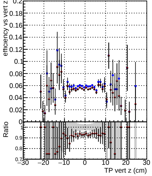
Efficiency —●— DQM_CKF_softQCD —●— DQM_mkFit_softQCD —●— DQM_mkFit_softQCD-newTr2
