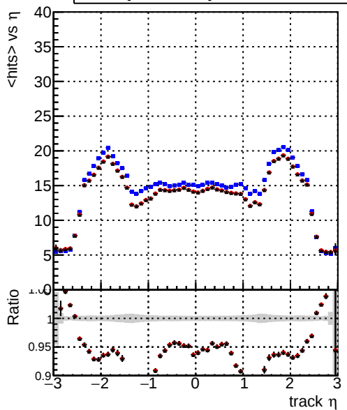
— DQM_CKF_softQCD — DQM_mkFit_softQCD — DQM_mkFit_softQCD-newTr2 mean hits
