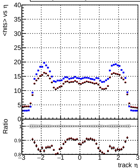
— DQM_CKF_softQCD — DQM_mkFit_softQCD — DQM_mkFit_softQCD-newTr2 mean hits
