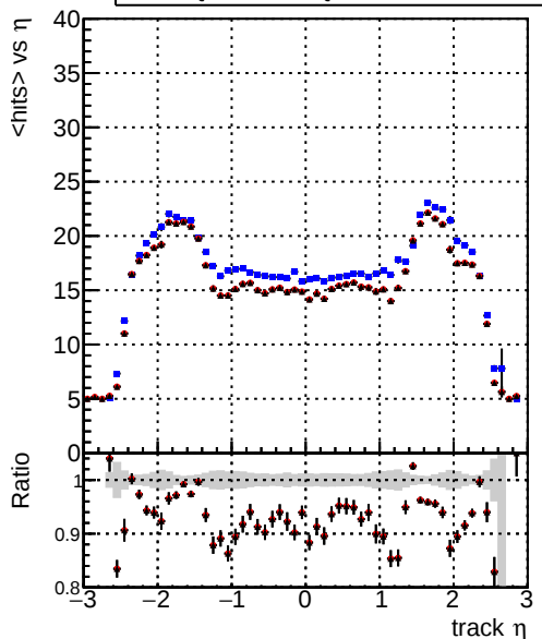
mean hits vs \eta — DQM_CKF_softQCD — DQM_mkFit_softQCD — DQM_mkFit_softQCD-newTr2
