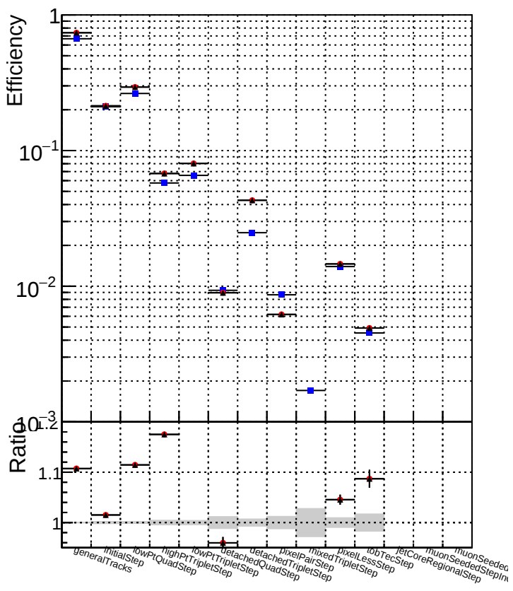
DQM_CKF_softQCD DQM_mkFit_softQCD DQM_mkFit_softQCD-newTr
