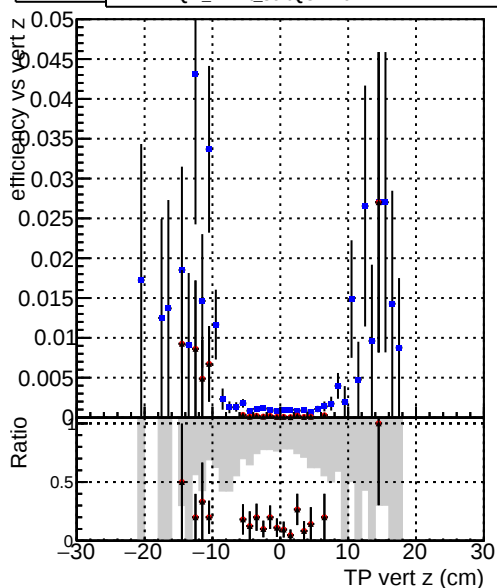
Efficiend —●— DQM_mkFit_softQCD —▲— DQM_mkFit_softQCD-newTr
