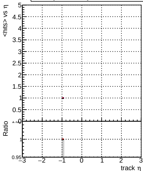
mean hits DQM_CKF_softQCD DQM_mkFit_softQCD DQM_mkFit_softQCD-newTr
