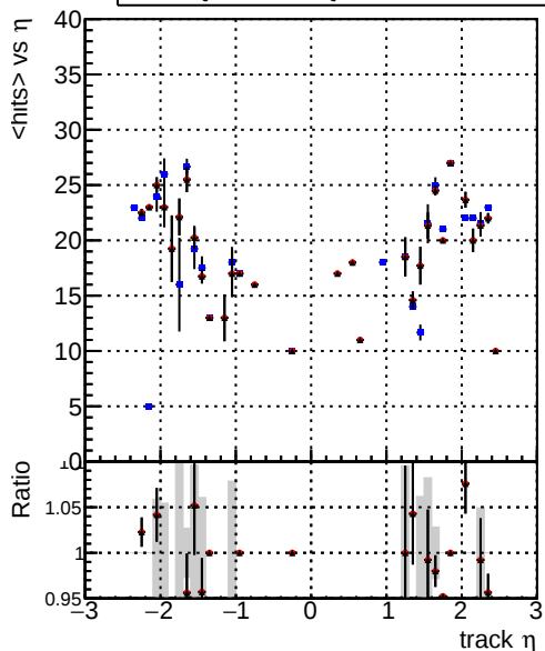
mean hit — DQM_ckpt_fit_softQCD — DQM_mkFit_softQCD — DQM_ckpt_fit_softQCD-newTr
