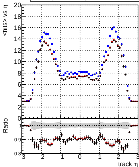
mean hit — DQM_CKF_softQCD — DQM_mkFit_softQCD — DQM_mkFit_softQCD-newTr
