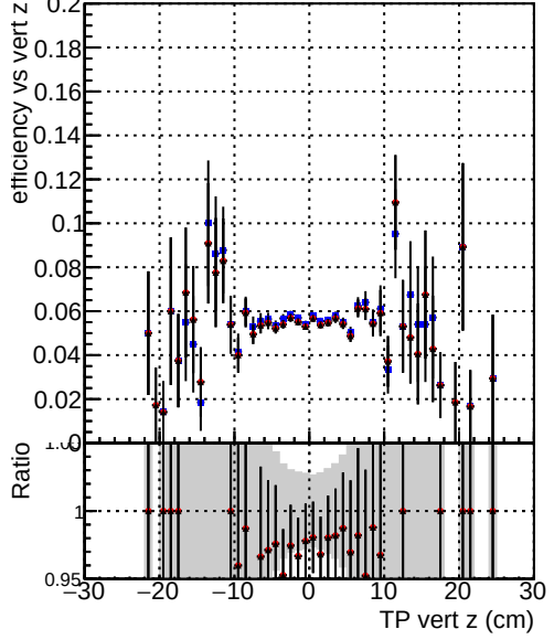
Efficiency vs. TP vert z (cm) —•— DQM_CKF_softQCD —•— DQM_mkFit_softQCD —•— DQM_mkFit_softQCD-newTr
