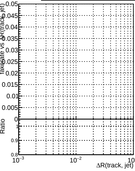
Fake rate vs \Delta R(\text{track}, \text{jet}) DQM_CKF_softQCD DQM_mkFit_softQCD DQM_mkFit_softQCD-newTr
