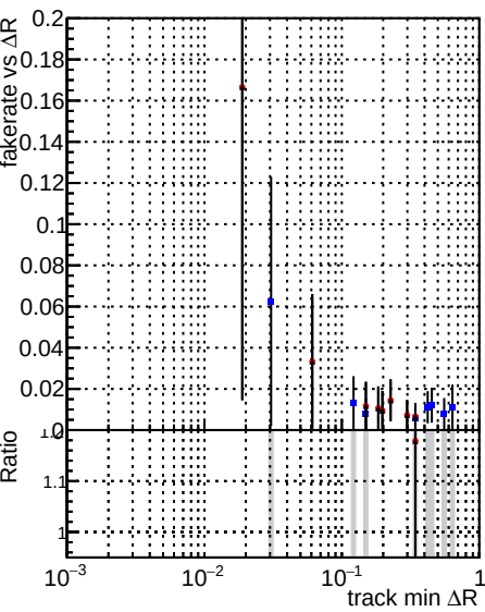
Legend: DQM_CKF_softQCD (blue dot), DQM_mkFit_softQCD (red dot), DQM_mkFit_softQCD-newTr (black dot)
