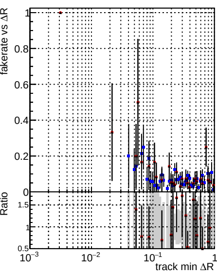
Fake rate vs \Delta R(\text{track, jet}) DQM_CKF_softQCD DQM_mkFit_softQCD DQM_mkFit_softQCD-newTr
