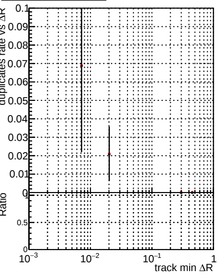
Legend: DQM_CKF_softQCD (blue circles), DQM_mkFit_softQCD (red circles), DQM_mkFit_softQCD-newTr (black circles)
