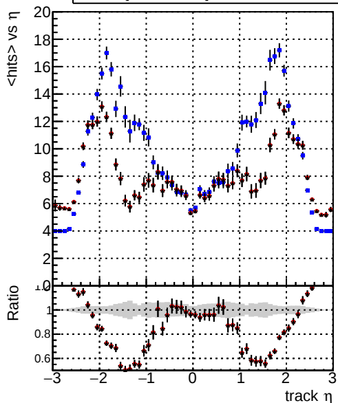
mean hits vs \eta — DQM_CKF_softQCD — DQM_mkFit_softQCD — DQM_mkFit_softQCD-newTr
