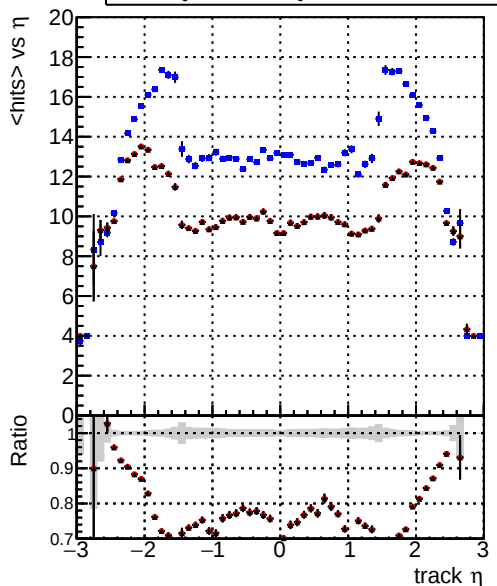
mean hit — DQM_CKF_softQCD — DQM_mkFit_softQCD — DQM_mkFit_softQCD-newTr
