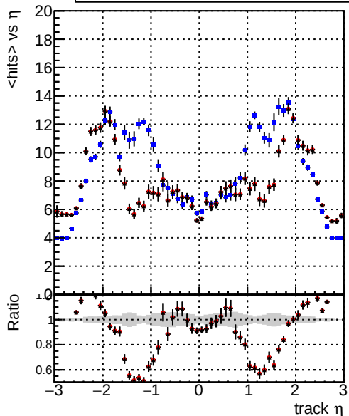
mean hit — DQM_CKF_softQCD — DQM_mkFit_softQCD — DQM_mkFit_softQCD-newTr
