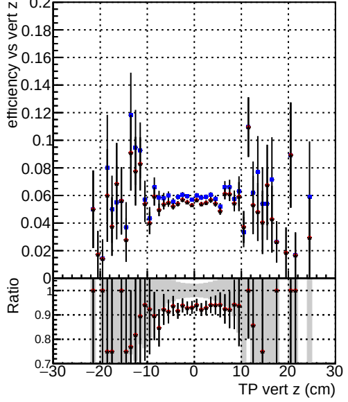
Efficiency —●— DQM_CKF_softQCD —●— DQM_mkFit_softQCD —●— DQM_mkFit_softQCD-newTr
