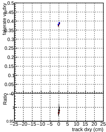
Legend: DOM CKE TTbarPU DOM CKE TTbarPU-noDNN3 DOM mktFit TTbarPU-clonerfix3
