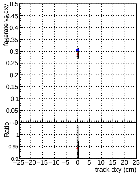
—•— DOM CKE TTbarPU —•— DOM CKE TTbarPU-noDNN3 —•— DOM mktFit TTbarPU-clonerfix3
