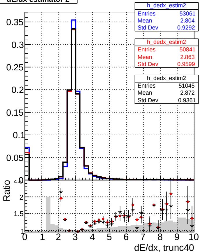
dE/dx estimator 2
