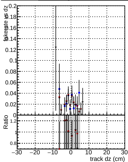
—•— DOM CKE TTbarPU —•— DOM mklfit TTbarPU-noDNN3 —•— DOM mklfit TTbarPU-clonerfix3
