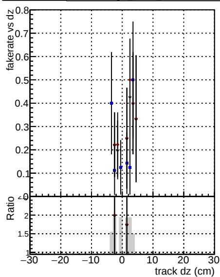
—•— DOM CKF TTbarPU —•— DOM CKF TTbarPU-noDNN3 —•— DOM mktFit TTbarPU-clonerfix3
