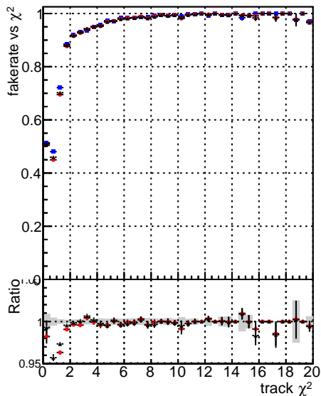
Fake rate vs. — BGM CKF TTbarPU — BGM mktFit TTbarPU-noDNN3 — BGM mktFit TTbarPU-clonerfix3
