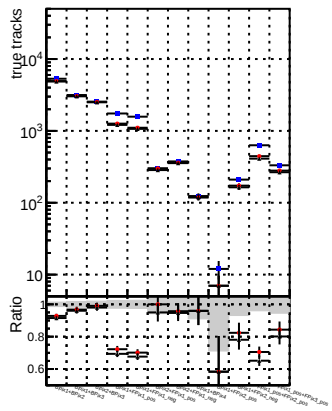
oDNN3 onertfix3
