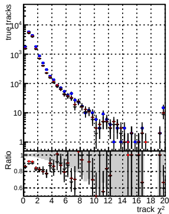
oDNN3 onertfix3
