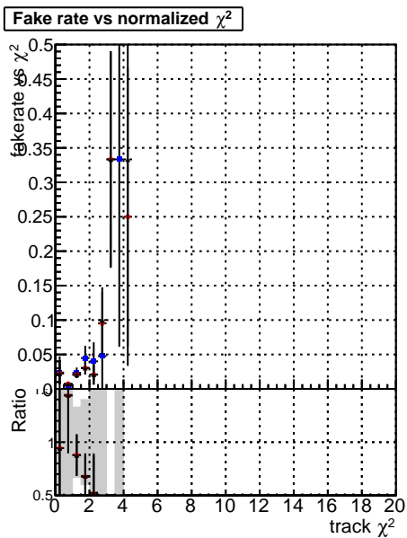
—•— DGM CKF TTbarPU —•— DGM CKF TTbarPU-noDNN3 —•— DGM CKF TTbarPU-clonerfix3
