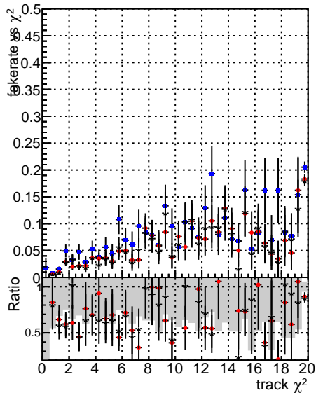
Fake rate vs. —●— DGM CKF TtbarPU —●— DGM mkFit TtbarPU-noDNN3 —●— DGM mkFit TtbarPU-clonerfix3
