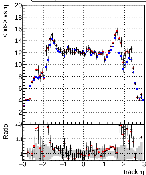
mean hits — DQM_CKF_TTbarPU — DQM_mkFit_TTbarPU — DQM_mkFit_TTbarPU-clonerfix2
