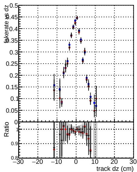
DOM CKE TTbarPU BOM mklfit TTbarPU-clonerfix2
