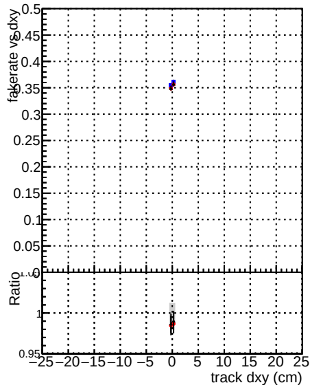
DOM CKE TTbarPU BOM mklfit TTbarPU-clonerfix2
